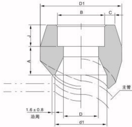
承插焊支管座 SW Outlets
